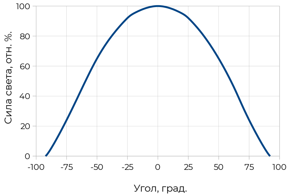
Кривая силы света (IF = 150мА, Tj = 25 °С)
