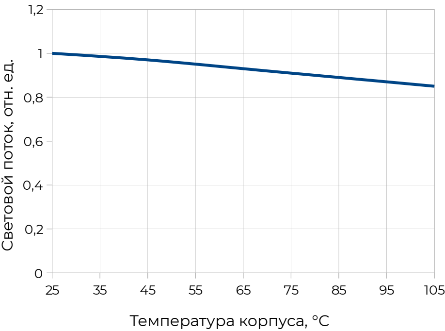
Зависимость светового потока от температуры перехода ( I_F = 150\text{мА} , T_j = 25\text{ °C} )
